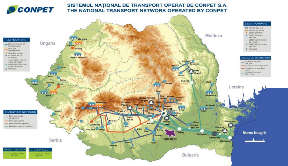
Grafic 16 - Sistemul național de transport operat de CONPET
